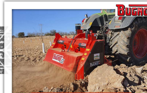
Trituradora BPM 2450
